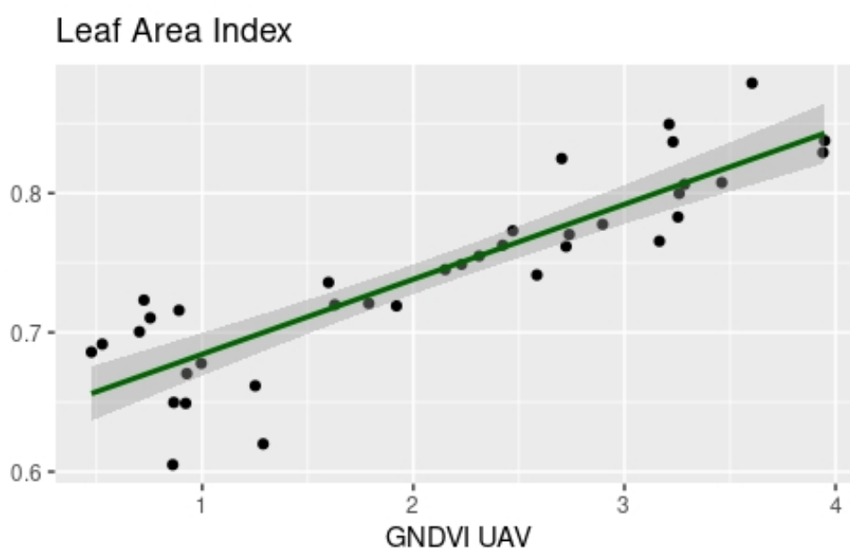
Figura 11. Correlazione tra la LAI e Gndvi rilevato dal drone
